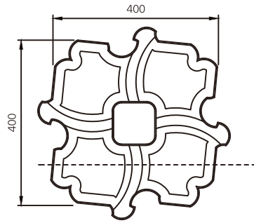
[ 평면도 ]
