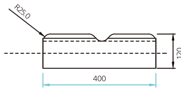
[ 정면도 ]
